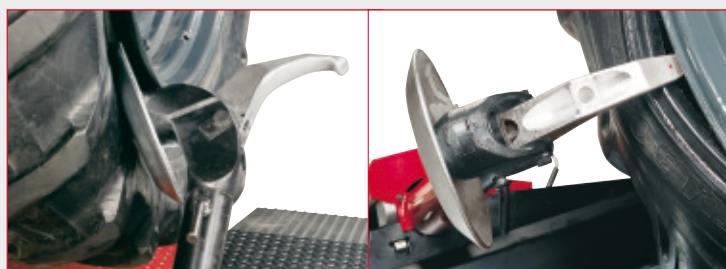
phase de détalonnage du pneu Abdruckphase
