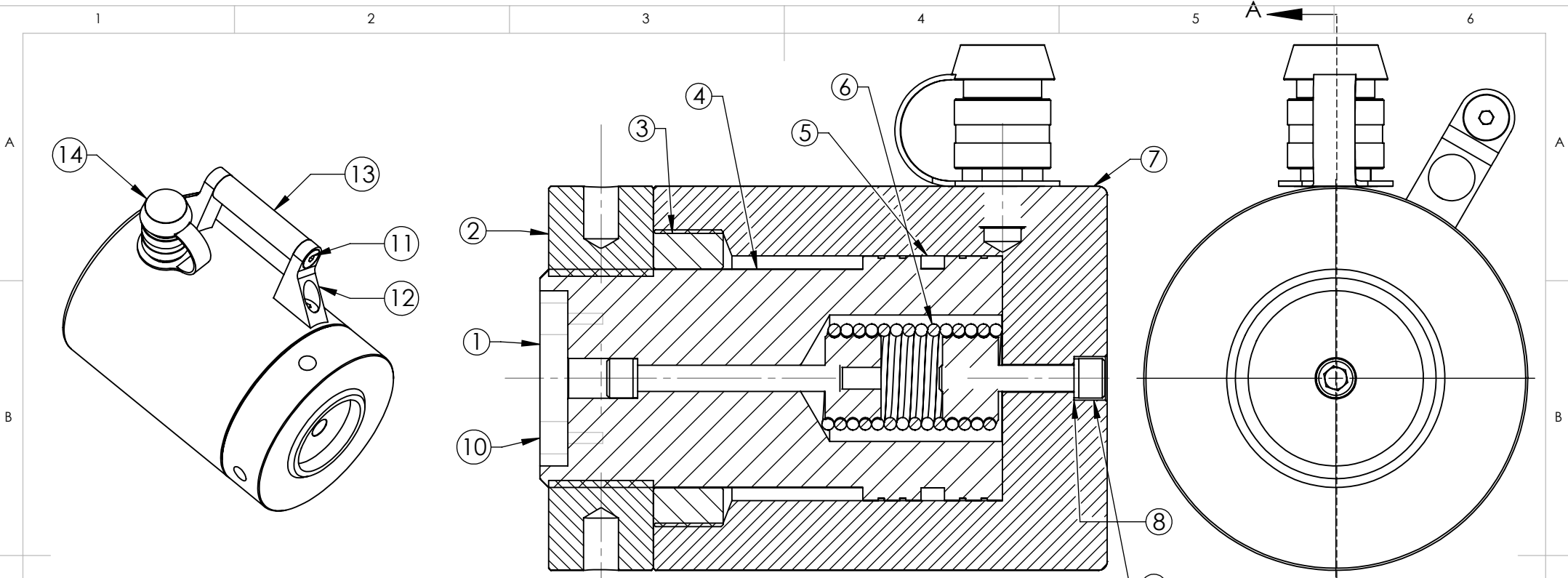
SECTION A-A
